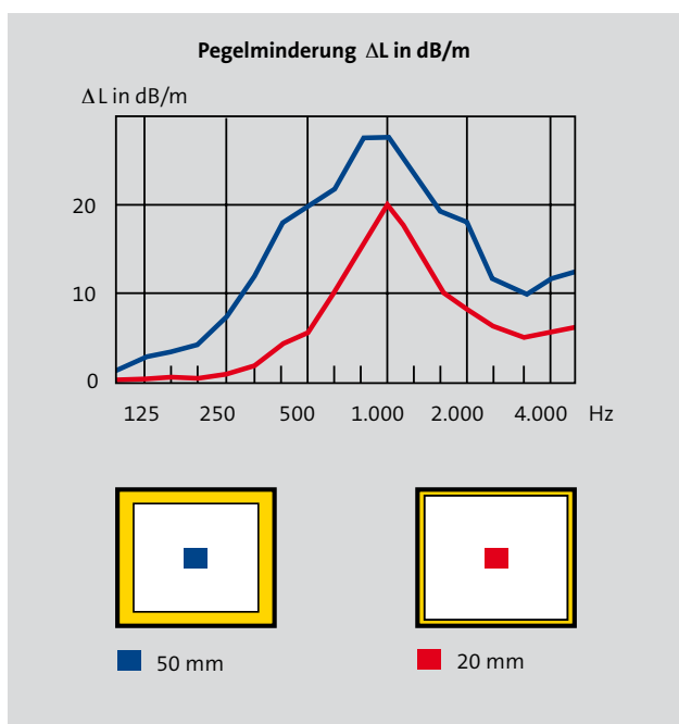
Pegelminderung schallabsorbierender Kanalauskleidungen
