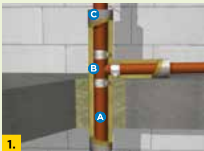
1. Abzweig mit U Protect Roll 3.1 Alu1
