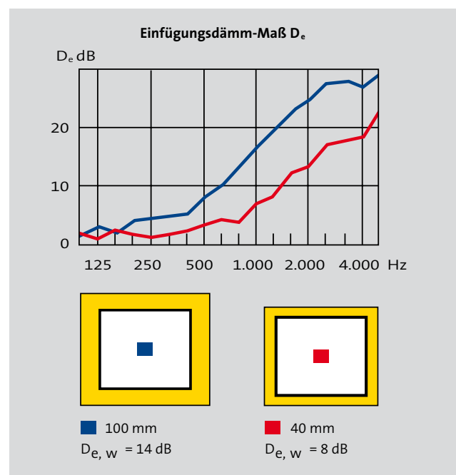
Einfügungsdämmung schalldämmender Kanalummantelungen
