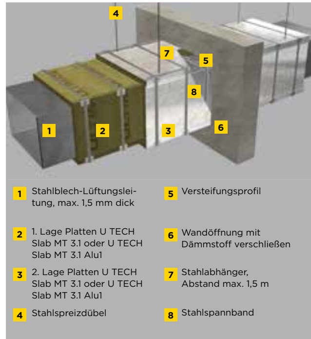
Waagerechte Lüftungsleitungen der Feuerwiderstandsklasse L30 bis max. 630 mm x 630 mm
