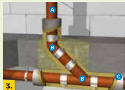
3. Sammelleitungsanschluss mit U Protect Roll 3.1 Alu1
