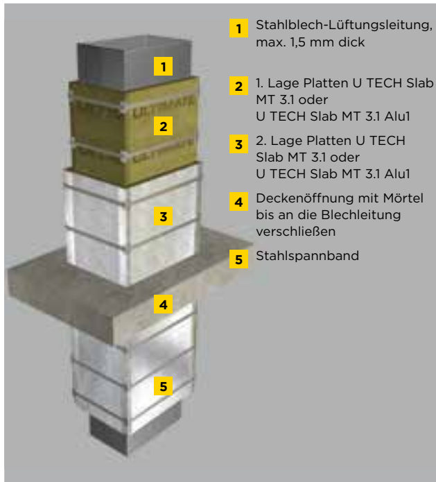
Senkrechte Lüftungsleitungen der Feuerwiderstandsklasse L30 bis max. 630 mm x 630 mm
