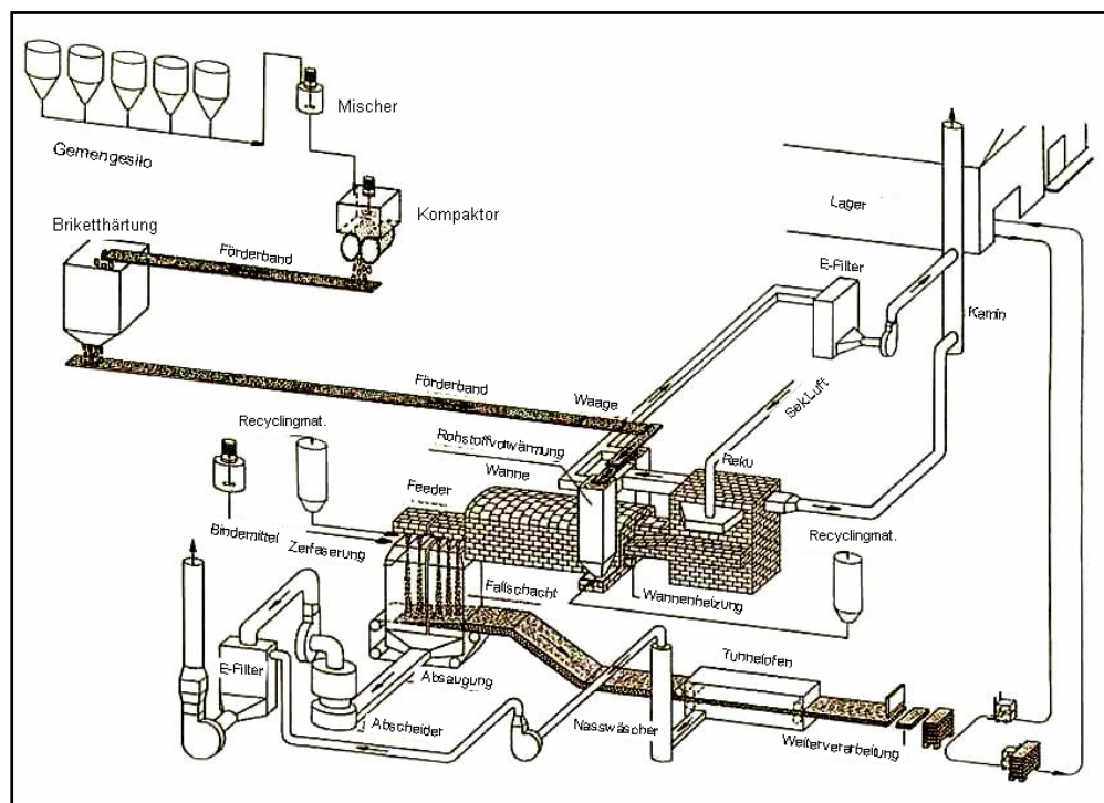
Abbildung 1: Prozessablauf
