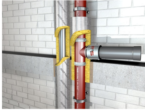
Bild 1: Die neue geprüfte Systemlösung von ISOVER und HES für den vorbeugenden Brandschutz bei Abwasser-Mischinstallationen macht Anschlüsse von Kunststoff-Abflussrohren an Abwasserleitungen aus Guss jetzt noch sicherer.
